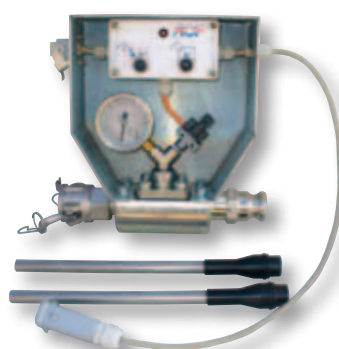
Kit "Spécial Injection"
