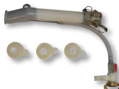
1 lance de projection + 3 buses à projeter Ø 8, Ø 12, Ø 16
